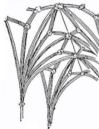
LIERNE VAULTING
