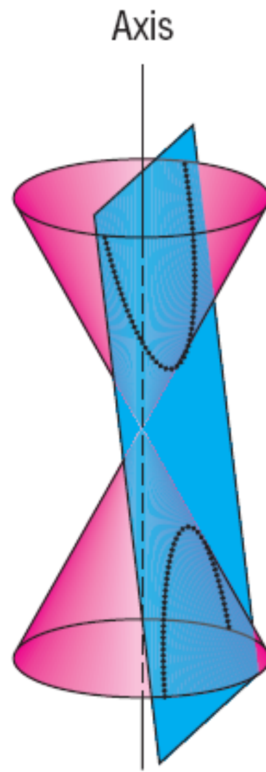
(d) Hyperbola
