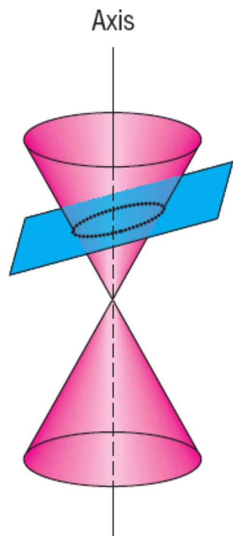
(b) Ellipse
